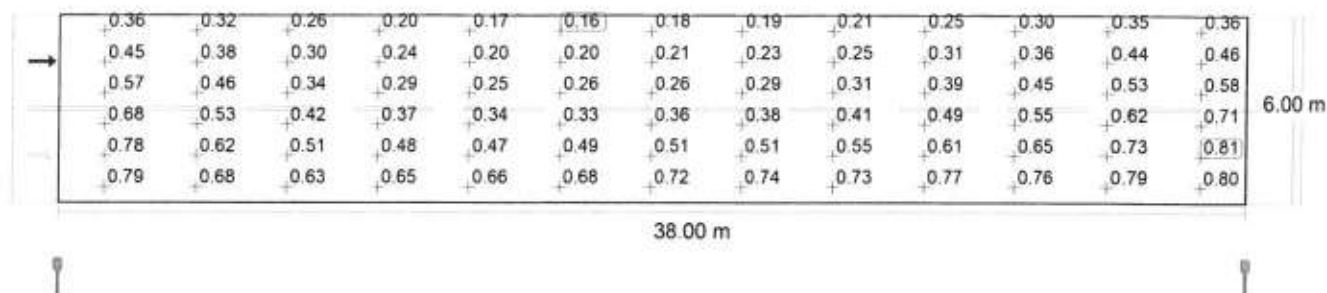
Observator 2: Densitatea luminii la instalația nouă [cd/m 2 ] (Raster valoric)
