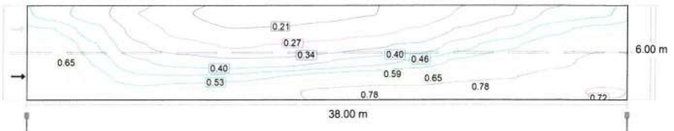
Observator 1: Densitatea luminii la instalația nouă [cd/m²] (Linii Isolux)
